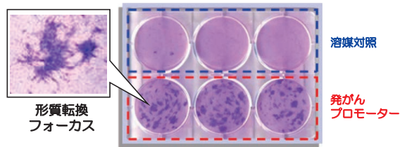
Bhas42細胞形質転換試験
