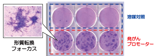
Bhas42細胞形質転換試験
