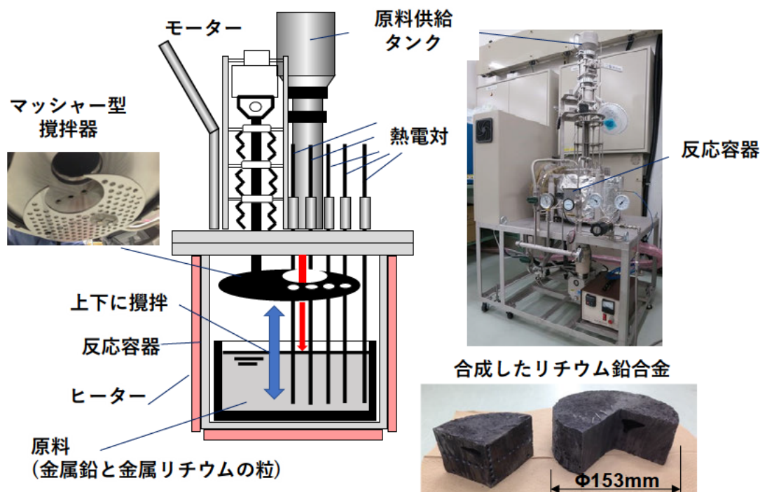
図 1 高純度リチウム鉛合金合成装置(量子科学技術研究開発機構との共同研究)
