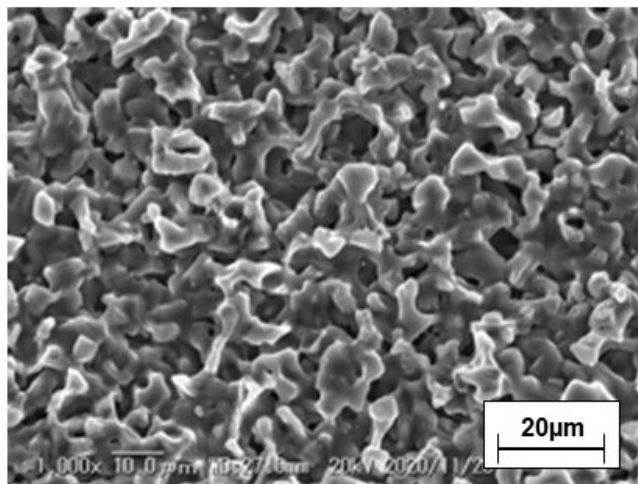
図2 液体金属中で優れた耐食性を示す FeCrAl 合金とその表面に形成される酸化被膜
